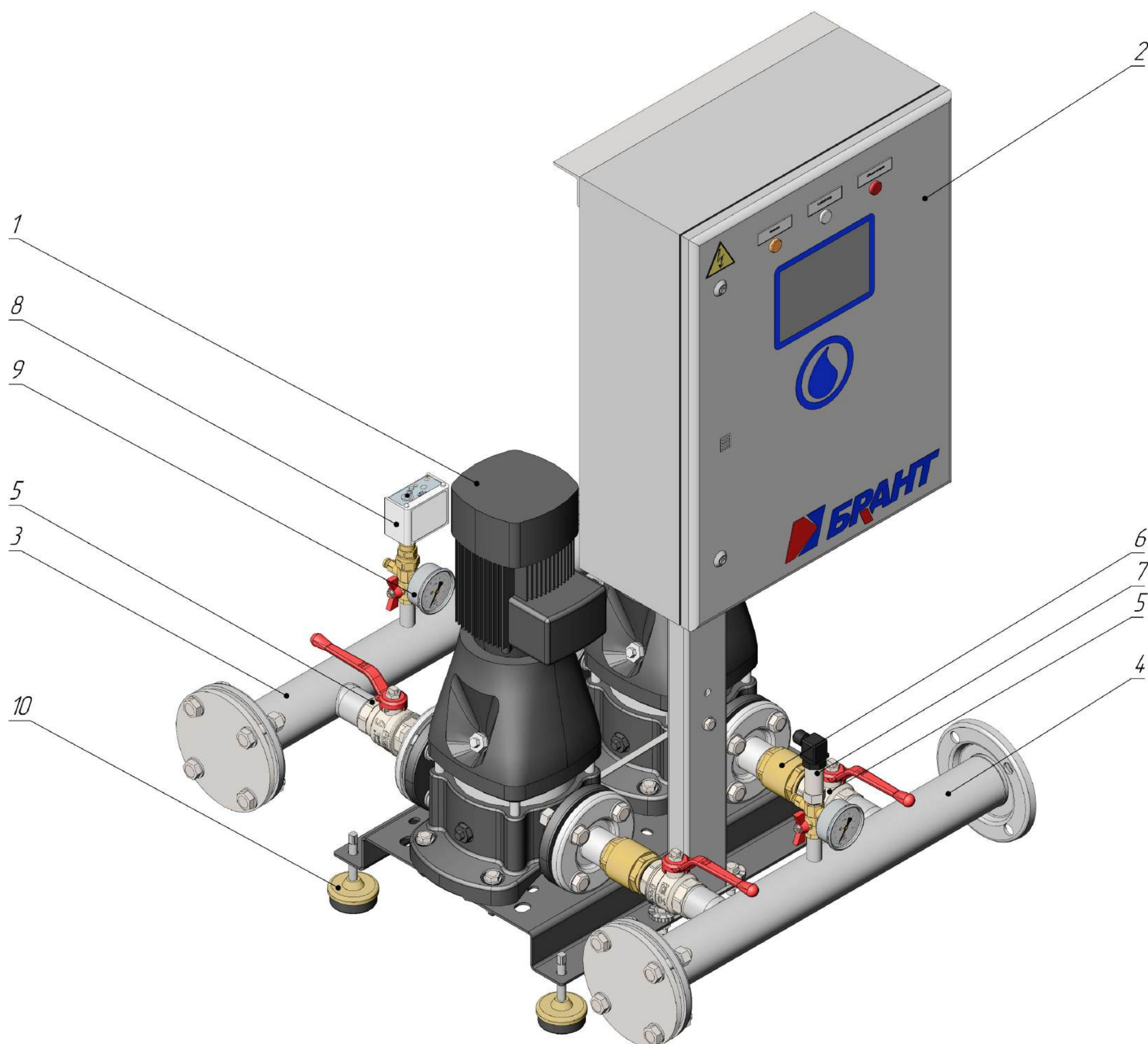
Рисунок – 15. Основное оборудование насосной установки серии Ч:
