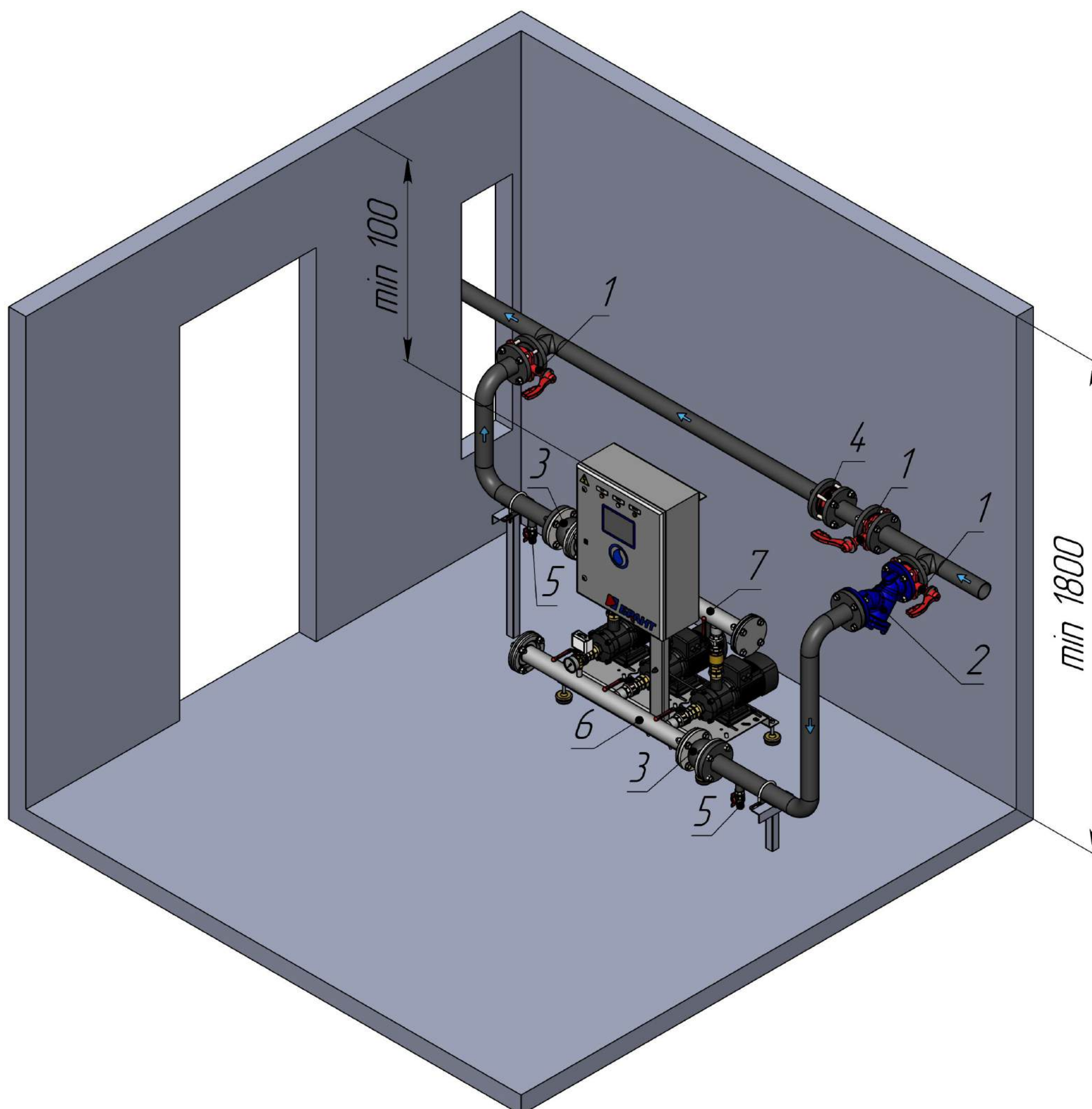
Рисунок – 10. Рекомендуемый вариант подключения насосной установки хозяйственно-питьевого водоснабжения к водопроводной сети с указанием рекомендуемой высоты помещения насосной станции:
