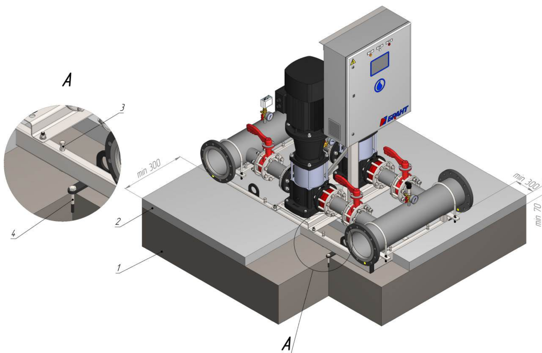
Рисунок – 12. Схема установки насосных установок с насосами мощностью более 11 кВт: 1 – фундамент, 2 – фиксирующая бетонная стяжка, 3 – нивелировочный болт, 4 – анкерный болт
