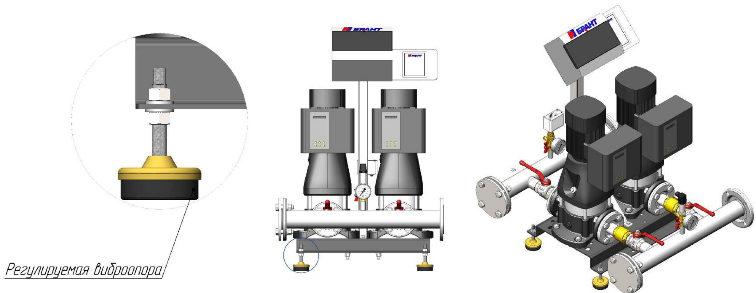
Рисунок – 11. Регулируемые виброопоры на насосной установке
