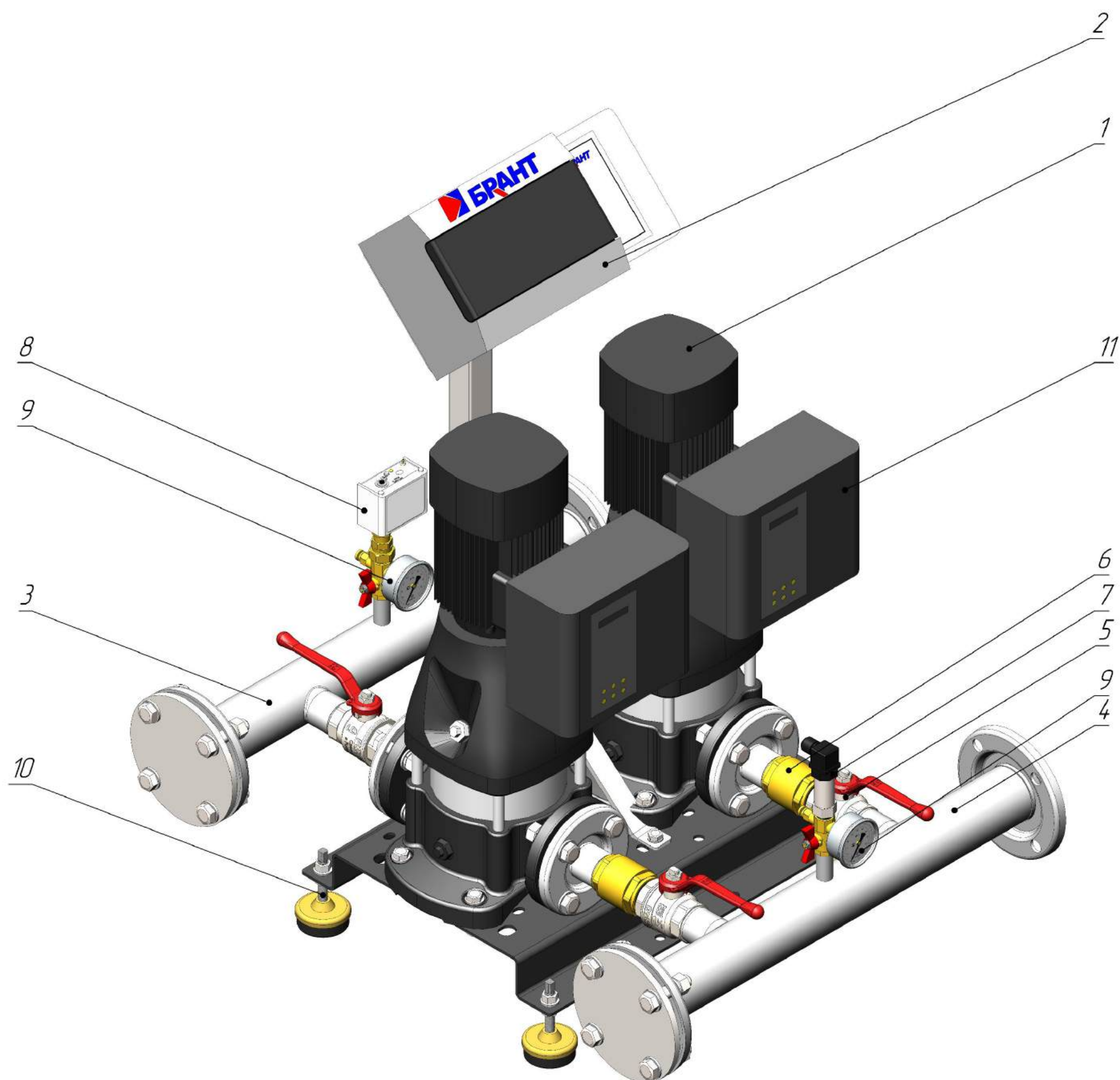
Рисунок – 16. Основное оборудование насосной установки серии ЧС:
